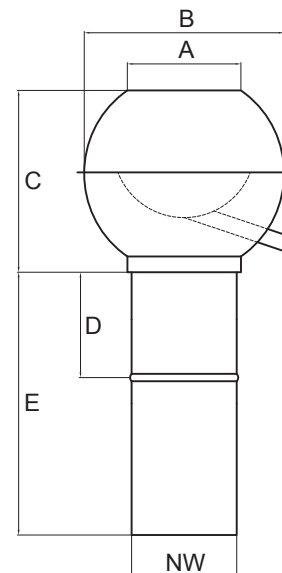
Typ POT mit Sicke und Standrohr 200 mm lang
