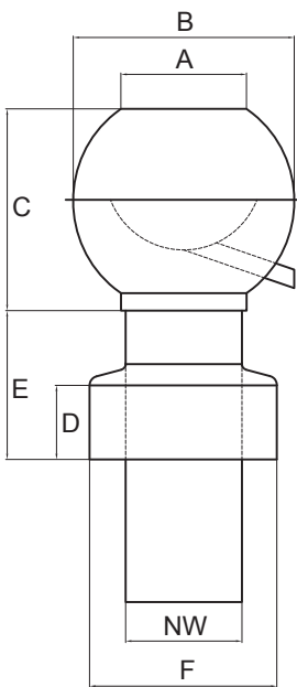
Typ PMT mit Abschlusstrichter und Standrohr 250 mm lang
