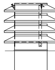
Typ ERB à section ronde avec tablette de 50 mm
