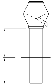
Typ ARID-F für Flachdach
