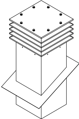
CE-S mit Tablett für Schrägdach
