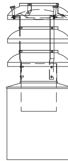
Type BM 500 à section ronde avec huisserie de fermeture longueur 500 mm
