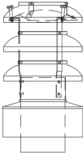
Type BM à section ronde avec huisserie de fermeture longueur 100 mm
