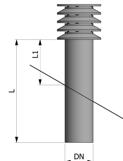
Type CRLD-S
