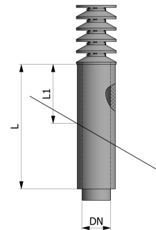
Type CRLD-S
