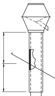
Tipo ARID-S per tetto a falda
