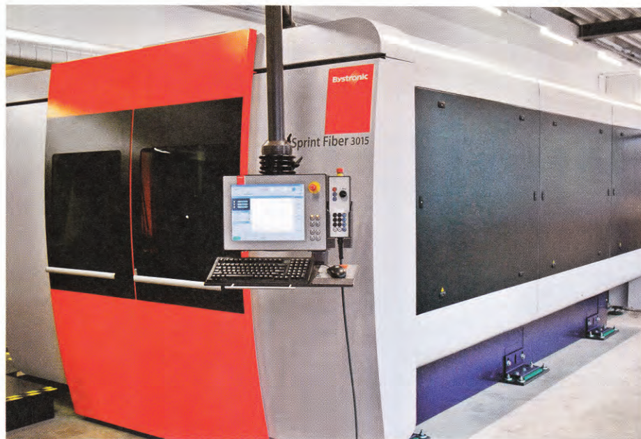
Le système de découpe laser BySprint Fiber 3015.
