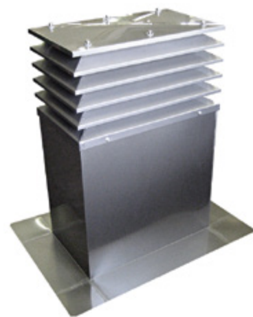
Castor CRLD/CEID-F: Aussenluft-Fassung, rund/eckig, Schutzgitter aus Cr-Ni-Stahl, doppelwandig gedämmt.
